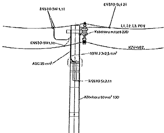
Bekötővezeték kialakítása és nullázás kialakítása (a lámpakar nullázása a védőösszekötő vezetõn)
