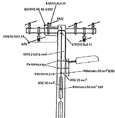
Bekötővezeték kialakítása és nullázás kialakítása (a lámpakar nullázása a védőösszekötő vezetõn)
