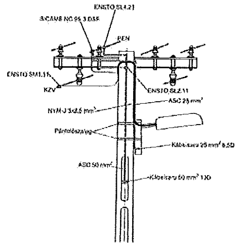
Bekötővezeték kialakítása és nullázás kialakítása (a lámpakar nullázása közvetlenül a PEN vezetõn)
